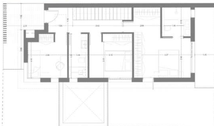
PRIMERA PLANTA
