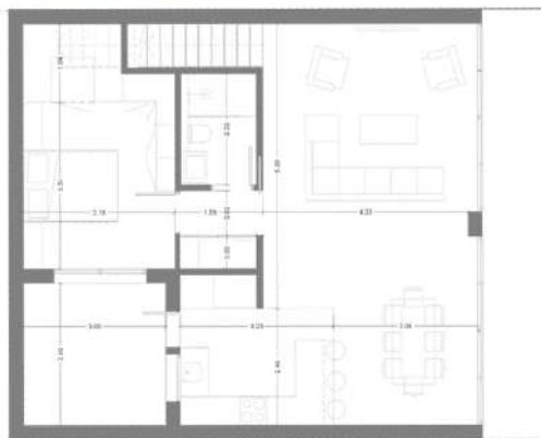
PLANTA BAJA
